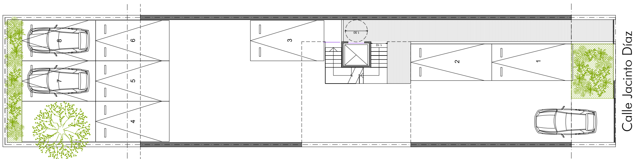
Planta Baja - Cocheras
