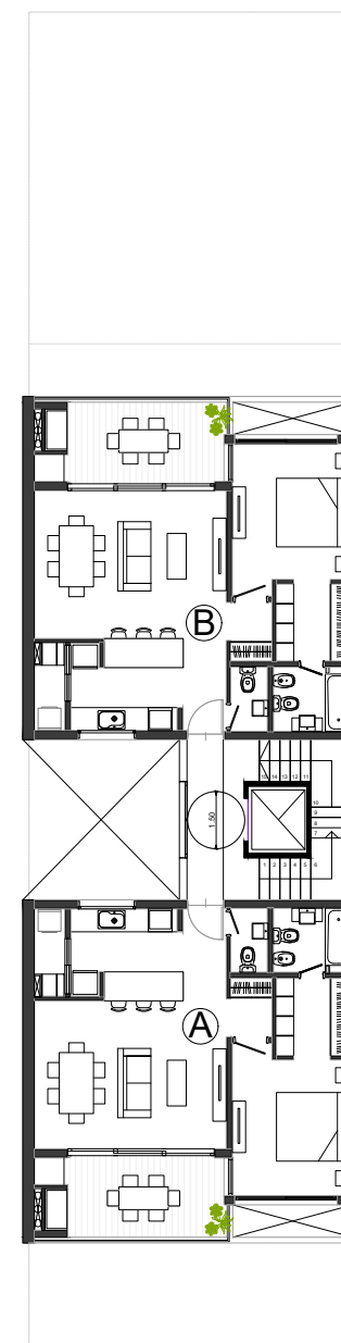
Planta Tipo
